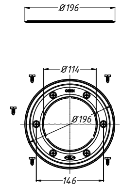
3. Обжимной фланец HL83.0
