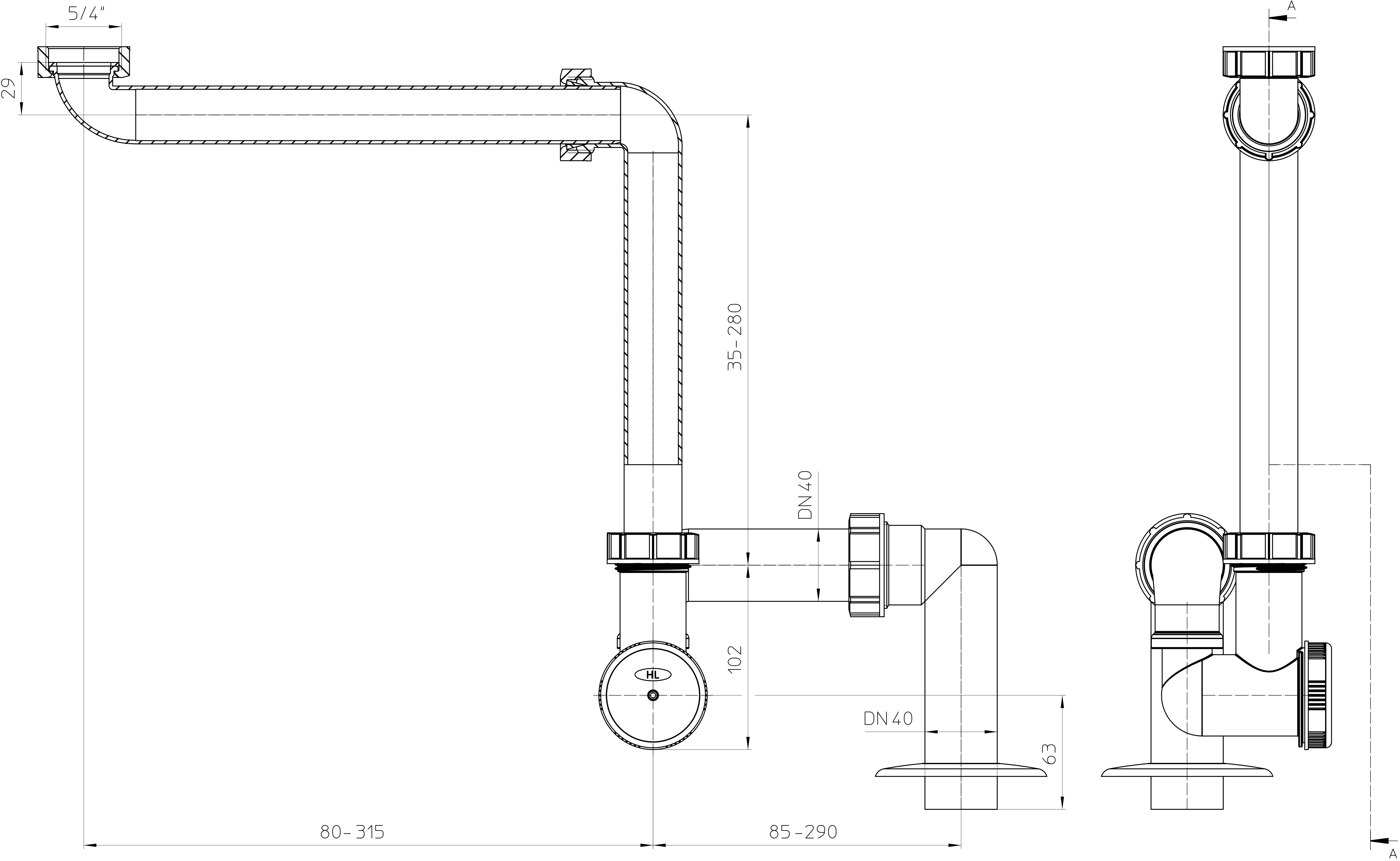
Schnitt A-A
