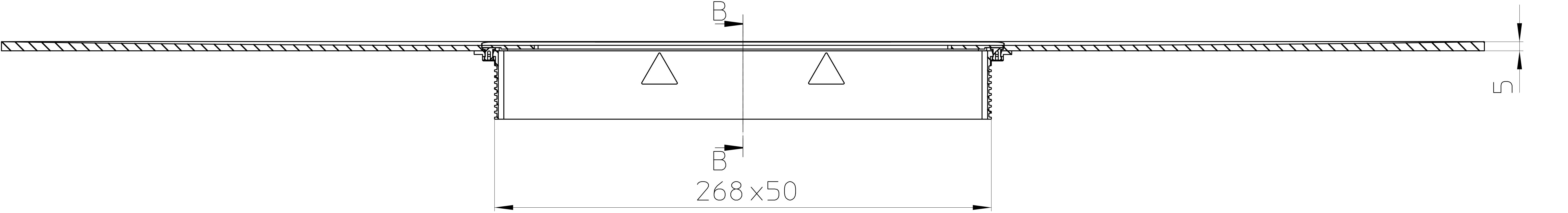
Schnitt A-A
