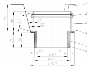
Рис. 6. Противопожарная муфта HL870 для кровельной воронки HL62.1/1.
