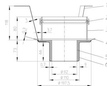
Рис. 5. Противопожарная муфта HL850 для кровельной воронки HL62.1/7.
