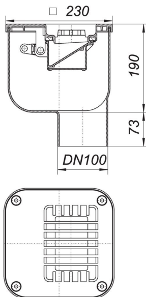
Рис.1. Трап HL680.
