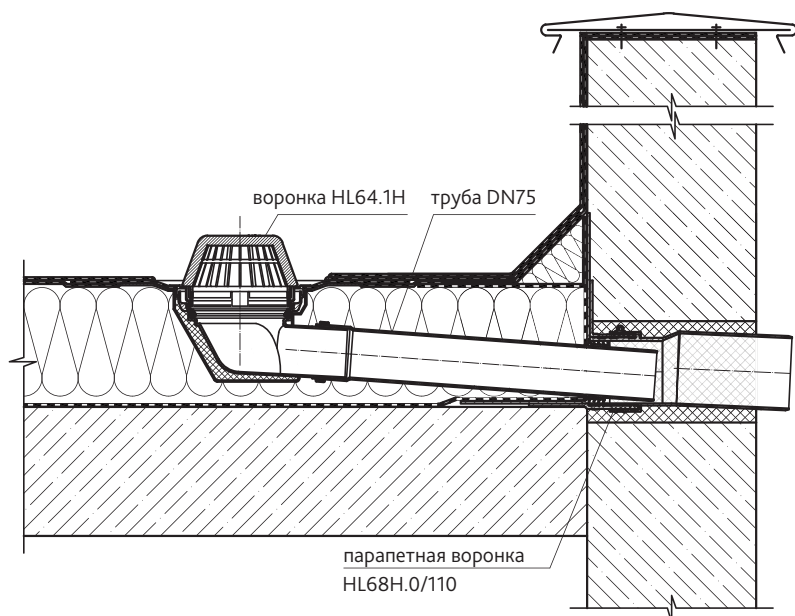
Применение кровельной воронки HL64.1H с парапетной воронкой HL68H.O/110
