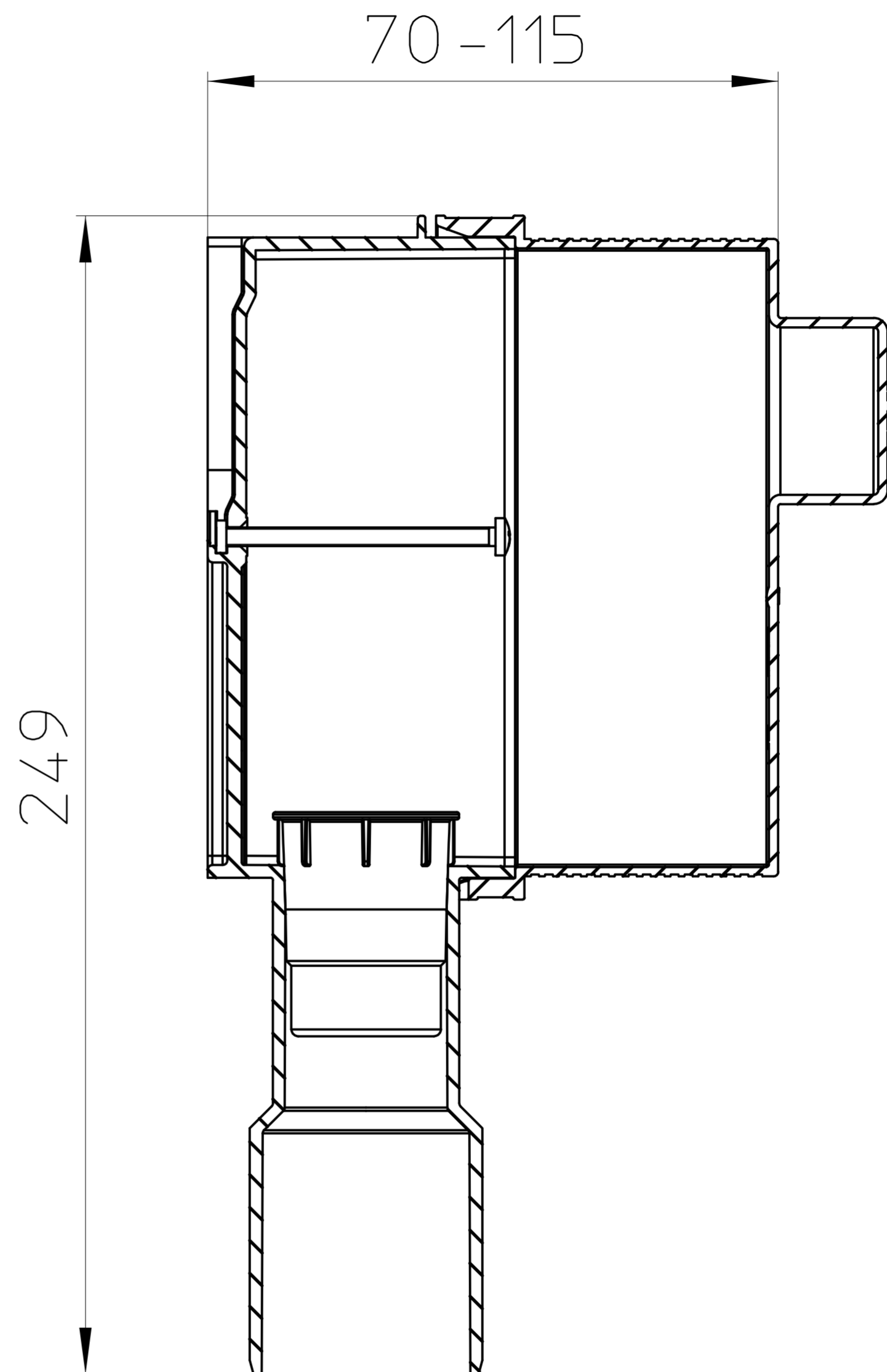
Schnitt A-A
