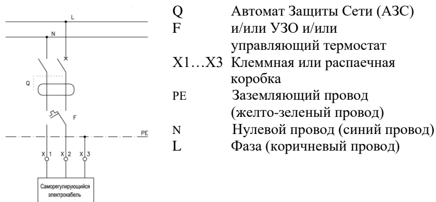
Рис. 2. Схема подключения электрообогрева кровельной воронки HL64.1Н к электрической сети.
