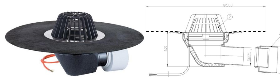
Рис. 1. Кровельная воронка с электрообогревом HL64.1Н
