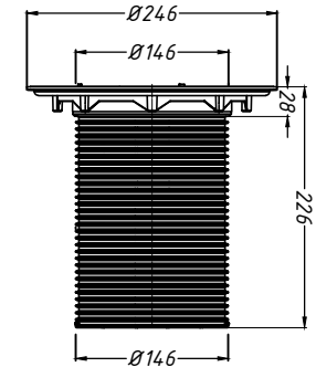
4. Наставной элемент с фланцем HL8500
