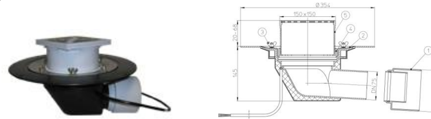
Рис. 1. Кровельная воронка HL64.1В
