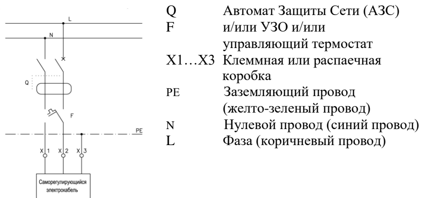
Рис. 2. Схема подключения электрообогрева кровельной воронки HL64.1 к электрической сети.
