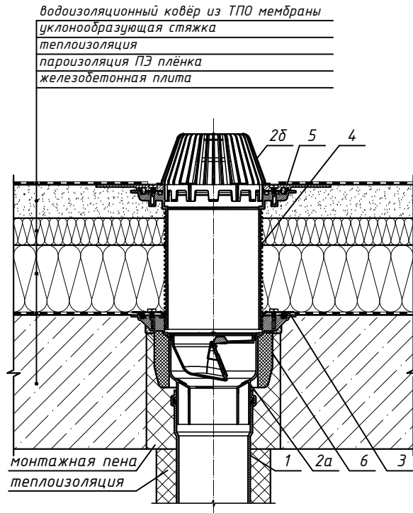
3. Обжимной фланец HL8300.0
