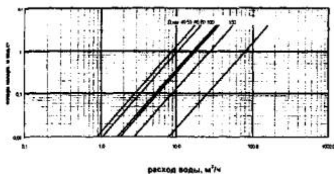
потери напора в турбинных счетчиках воды
