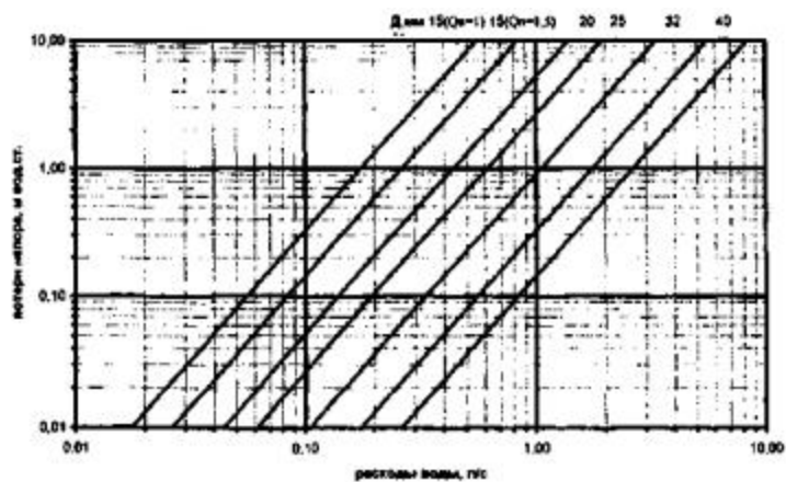
потери напора в турбинных счетчиках воды
