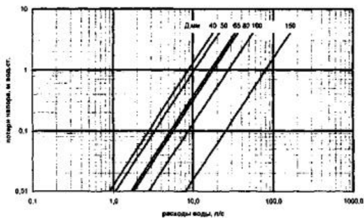
потери напора в турбинных счетчиках воды
