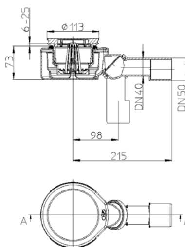
Schnitt A-A
