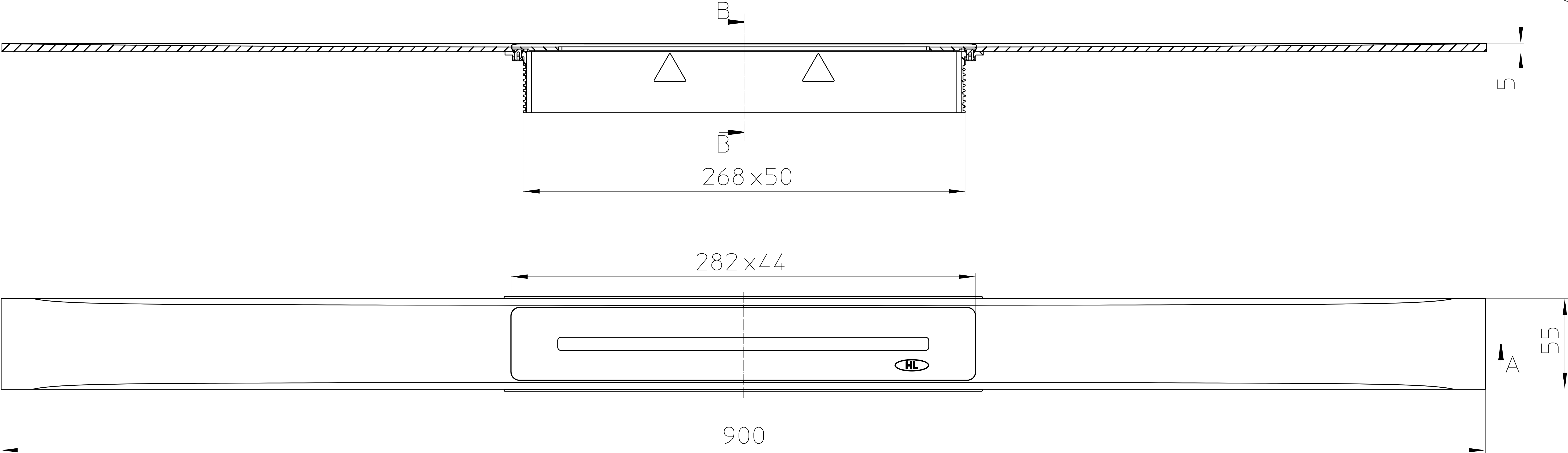
Schnitt A-A
