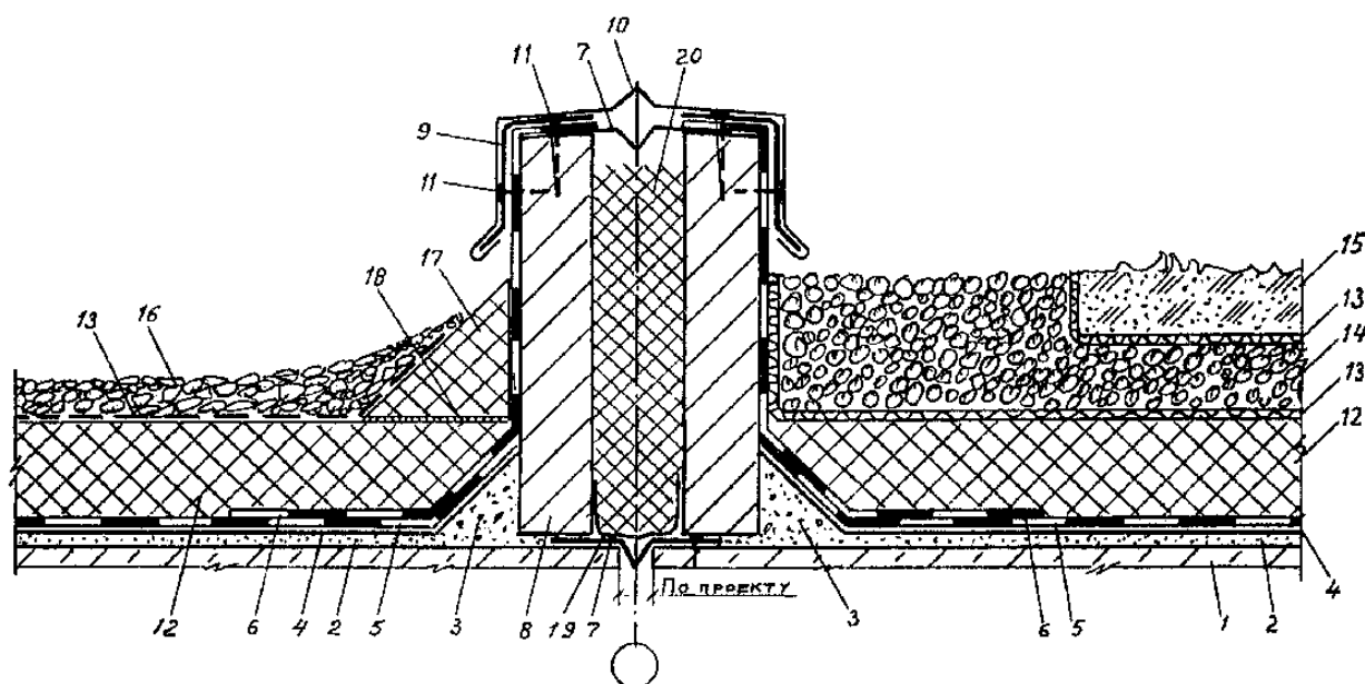
Рис. 6 Деформационный шов при инверсионной эксплуатируемой кровле.
