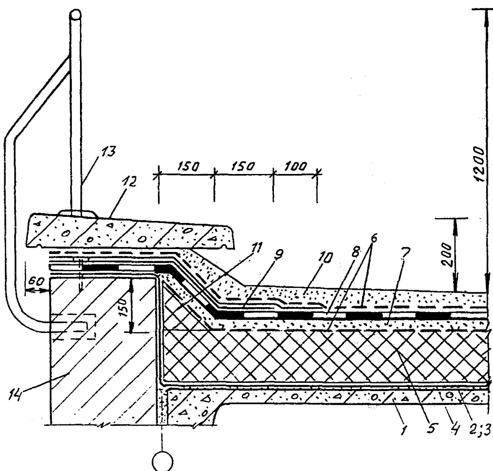
Рис. 7 Парапет продольной стены при традиционной эксплуатируемой кровле
