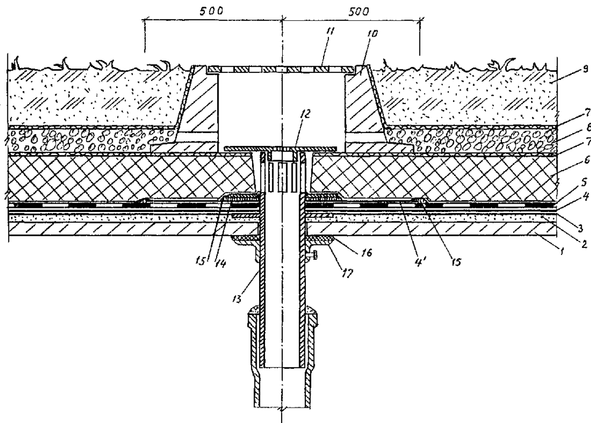
Рис. 11 Воронка внутреннего водостока при инверсионной эксплуатируемой кровле
