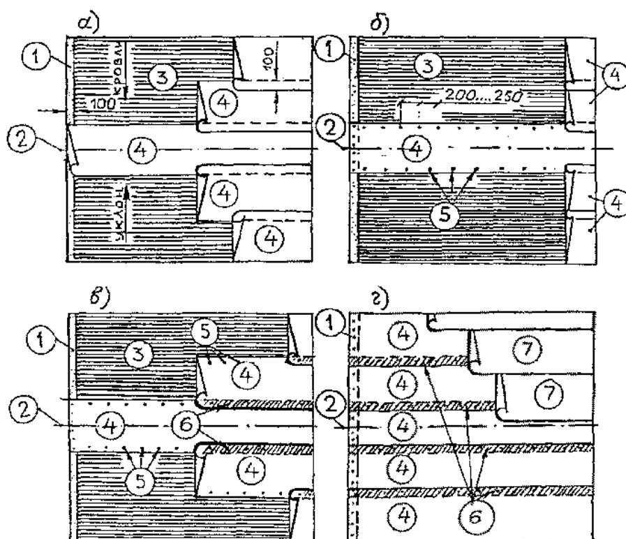
Рис. 1 Последовательность (а, б, в, г) раскладки рулонных материалов при устройстве водоизоляционного ковра с механическим закреплением нижнего слоя.
