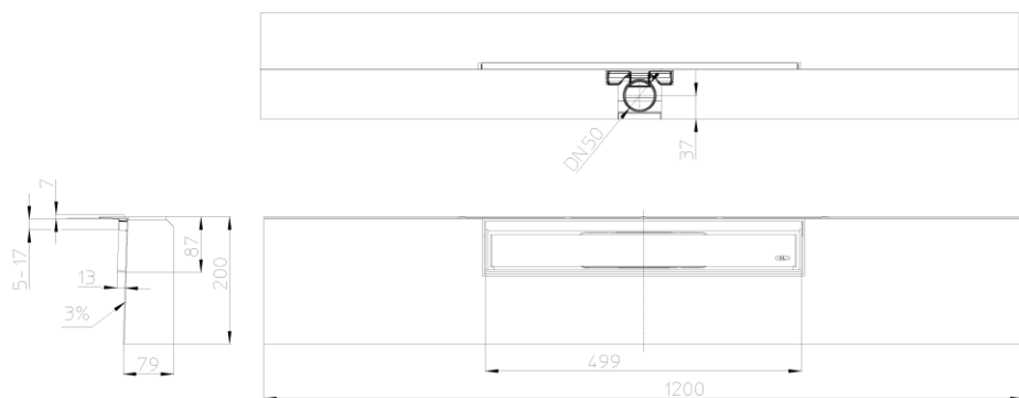
Рис. 1. Корпус лотка HL531
