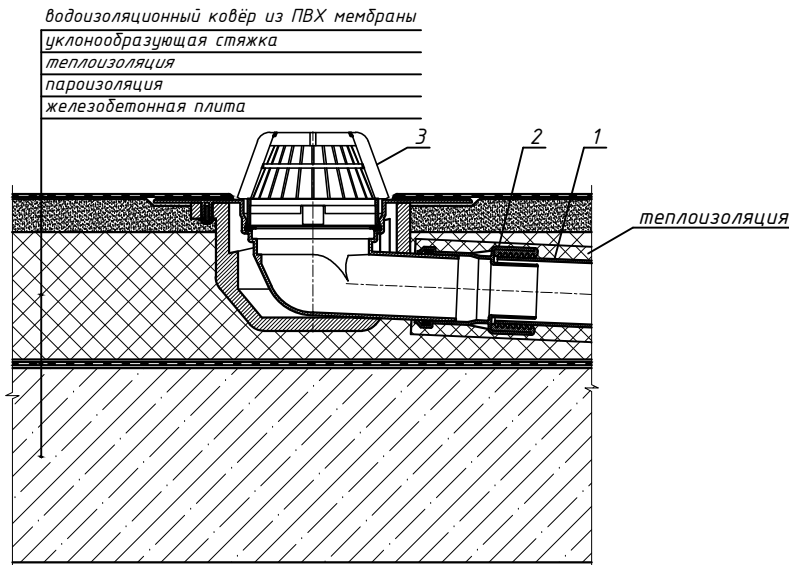
2. Переходник HL9/7
