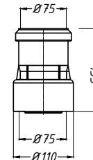
2. Переходник HL9/7
