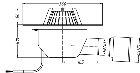
3. Воронка HL64.1P
