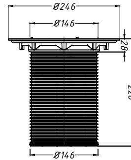
4. Надставной элемент с фланцем HL8500
