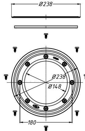
3. Обжимной фланец HL8300.0
