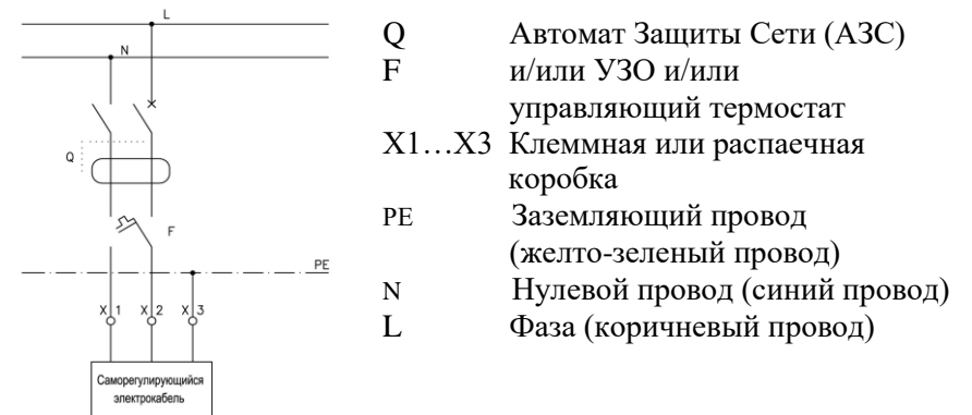
Рис. 3. Схема подключения электрообогрева кровельной воронки HL64.1BP к электрической сети.
