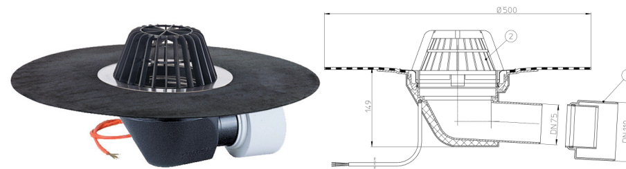
Рис. 1. Кровельная воронка с электрообогревом HL64.1Н
