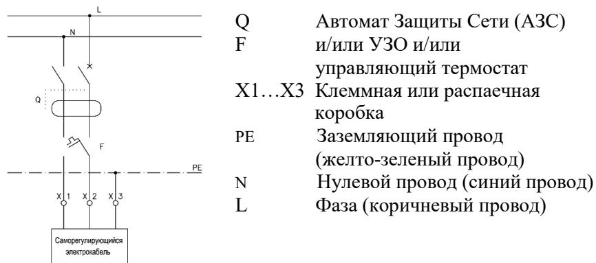
Рис. 2. Схема подключения электрообогрева кровельной воронки HL64.1Н к электрической сети.
