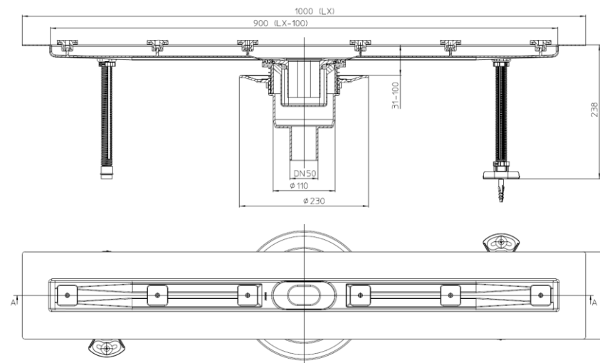
Рис. 1. Корпус лотка HL50FV.0/100.
