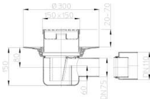
Рис.2. Трап HL72.1N.
