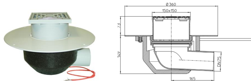
Рис. 1. Кровельная воронка HL64.1BP/7.
