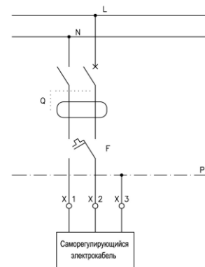
Рис. 3. Схема подключения электрообогрева кровельной воронки HL64.1BP/7 к электрической сети.
