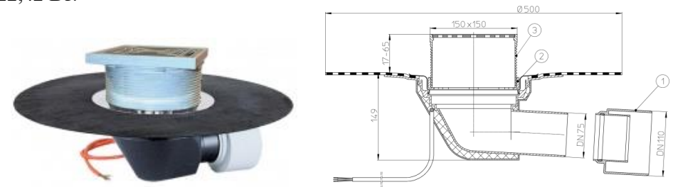
Рис. 1. Кровельная воронка с электрообогревом HL64.1BH
